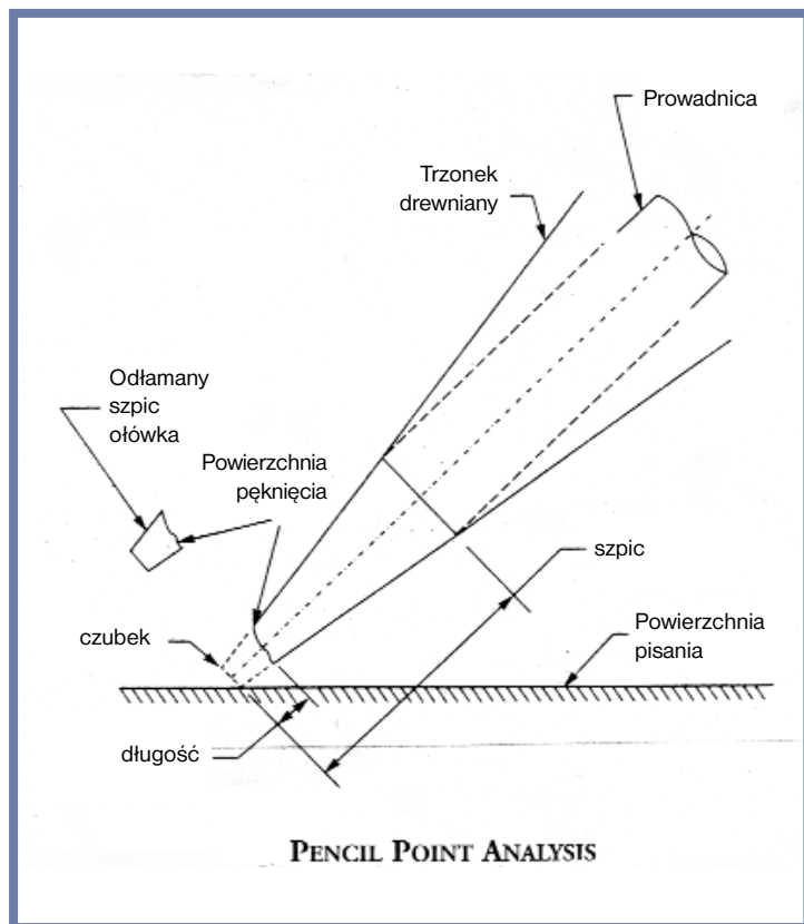
Analiza wytrzymałościowa szpica ołówka
